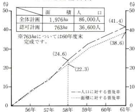
下水道整備計画
