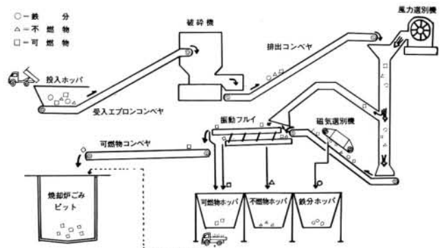
粗大ごみ破碎処理施設系統図
