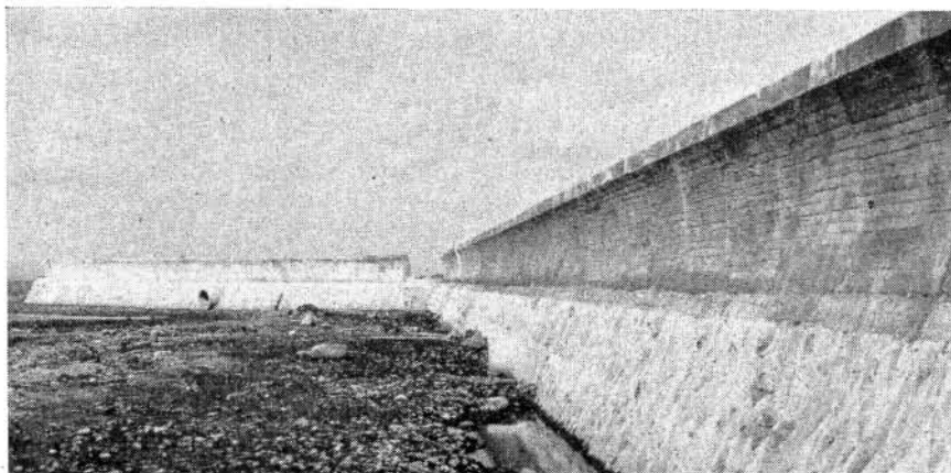
松山の海岸堤防ができあがりました。これは大村港海岸保全事業として行なわれたもので、長さ511メートル、高さ3.5メートルのものです。総工費1,800万円
