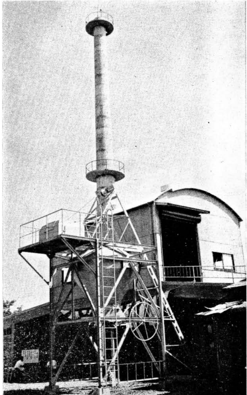
写真 — 新しくできた焼却炉
