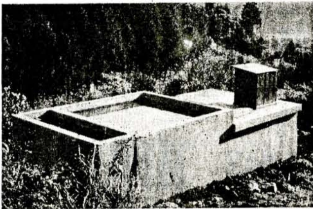
写真は上=三浦松の頭にできた共同防除施設(中央は貯水槽、右上は機械室)下=灌漑管無田の共同給水施設の貯水槽と浄化槽
