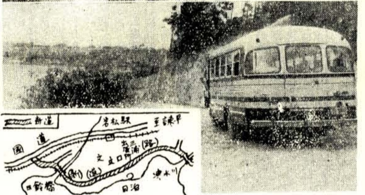
(写真(上)より三浦中學講堂・(中)は臨時バスが通つた三浦道路(下)は貝津―大村線略図)
