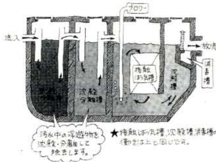
分離接触ばつ気方式
