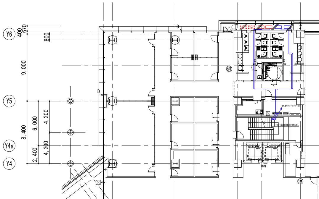
2階平面図
