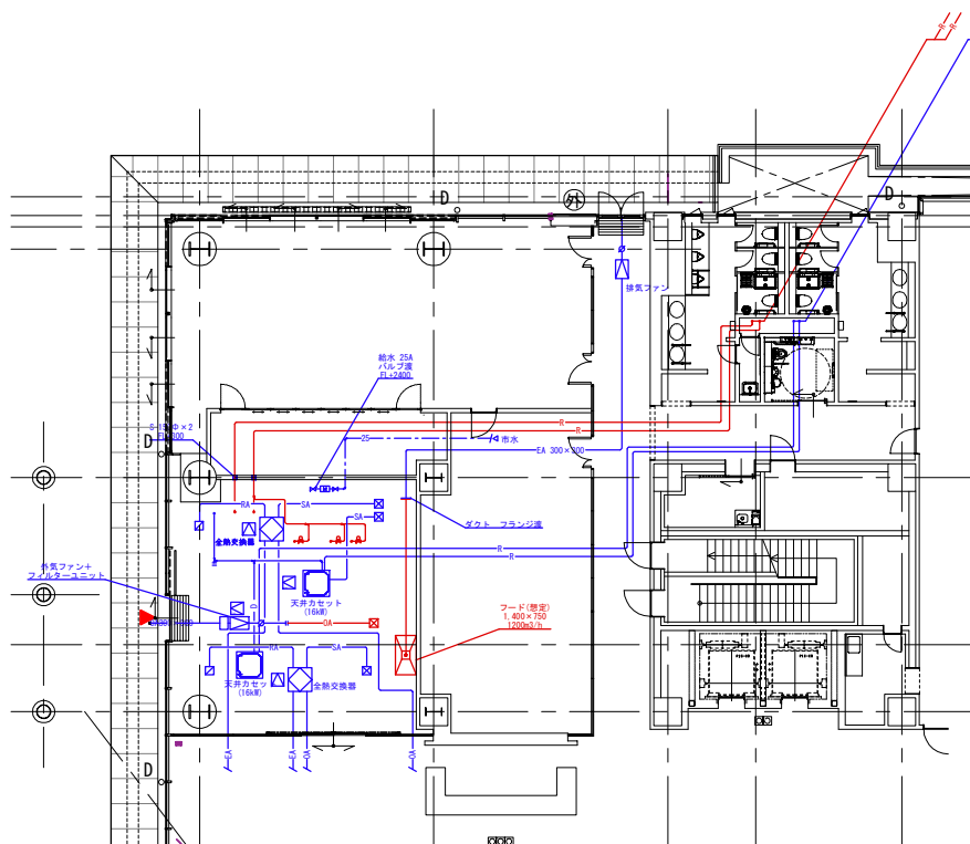
1階平面図(天井)
