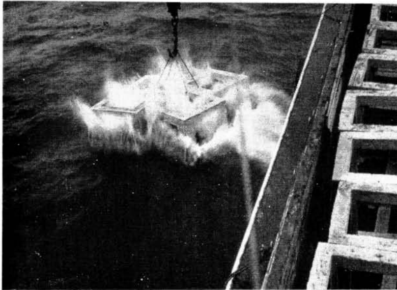
コンクリート漁罌の沈設作業
